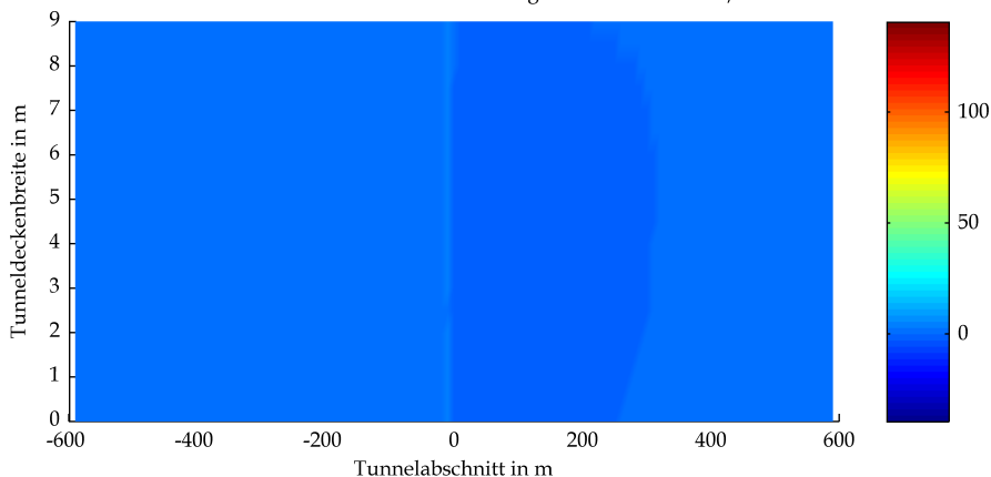
BAStBÜ Rechteck Mulde RV 20.6 owF Wärmestrahlung Tunneldecke in kW/m 2 bei t=3300s
