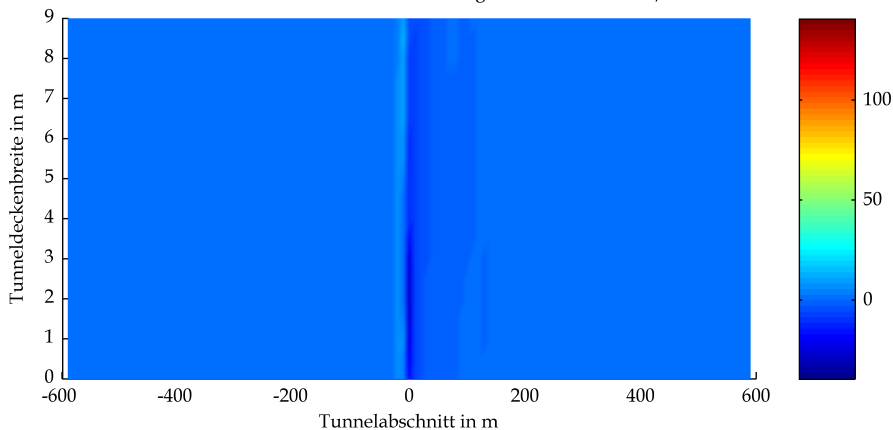
BAStBÜ Rechteck Mulde RV 20.6 owF Wärmestrahlung Tunneldecke in kW/m 2 bei t=2400s
