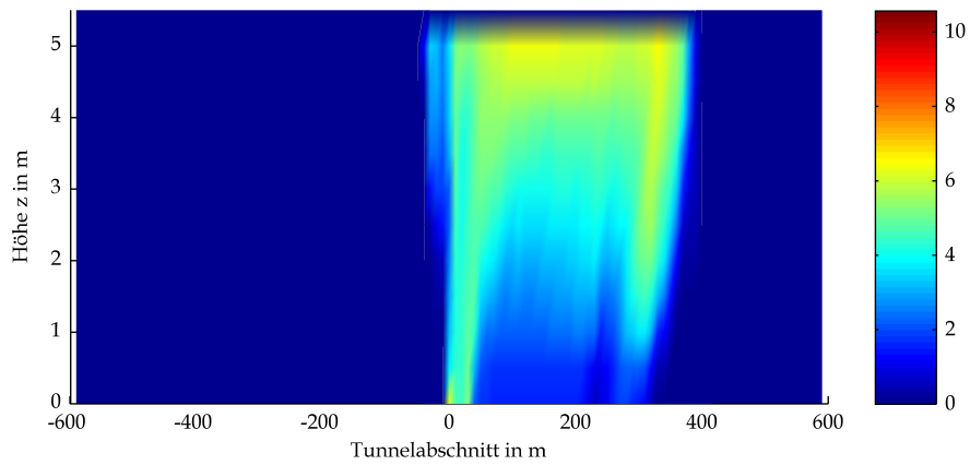
BASStBÜ Rechteck Mulde RV 20.6 owF Optische Dichte bei t=120s
