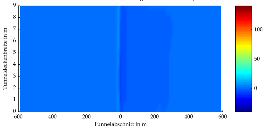
BAStBÜ Rechteck Mulde RV 20.6 owF Wärmestrahlung Tunneldecke in kW/m 2 bei t=3000s
