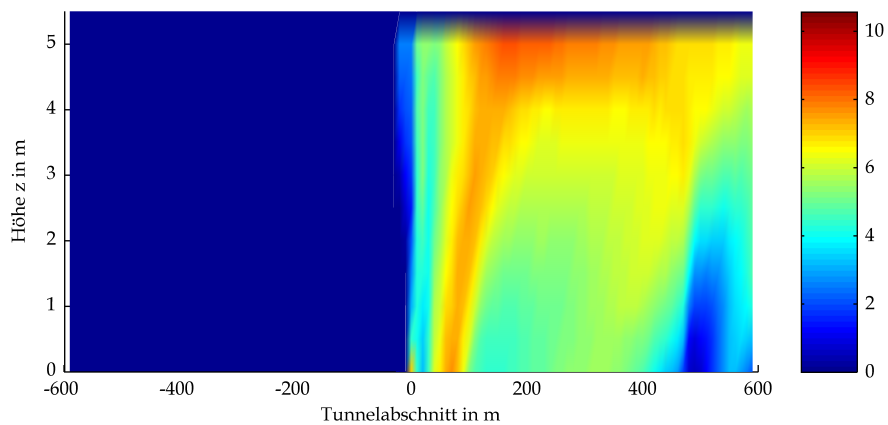
BASStBÜ Rechteck Mulde RV 20.6 owF Optische Dichte bei t=180s
