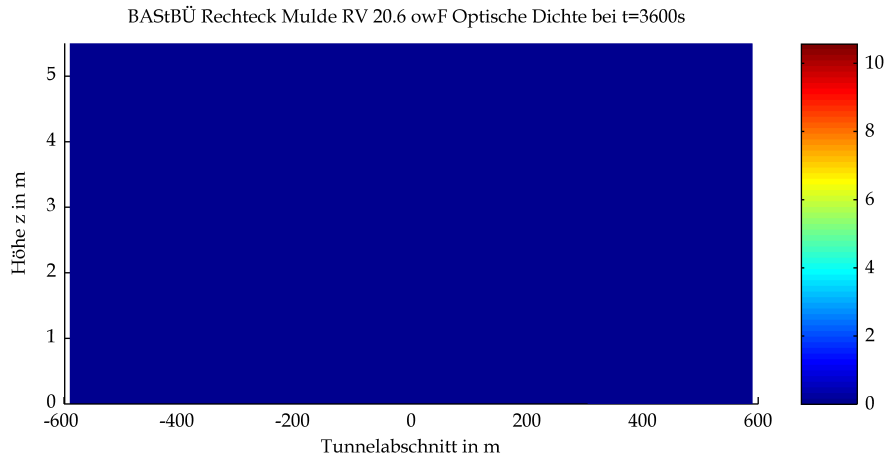
Mittels CFD-Berechnung ermittelte optische Dichten
