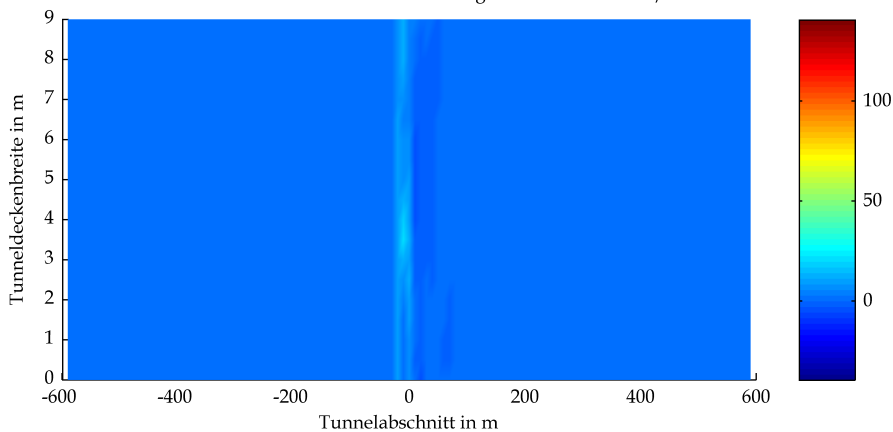
BAStBÜ Rechteck Mulde RV 20.6 owF Wärmestrahlung Tunneldecke in kW/m 2 bei t=2100s
