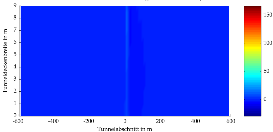
BAStBÜ Rechteck Mulde GV 20.6 owF Wärmestrahlung Tunneldecke in kW/m 2 bei t=3000s
