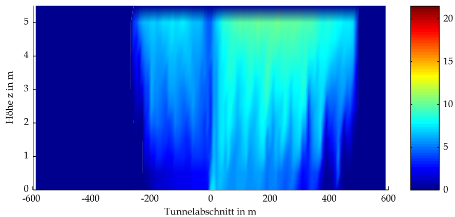
BAStBÜ Rechteck Mulde GV 20.6 owF Optische Dichte bei t=180s
