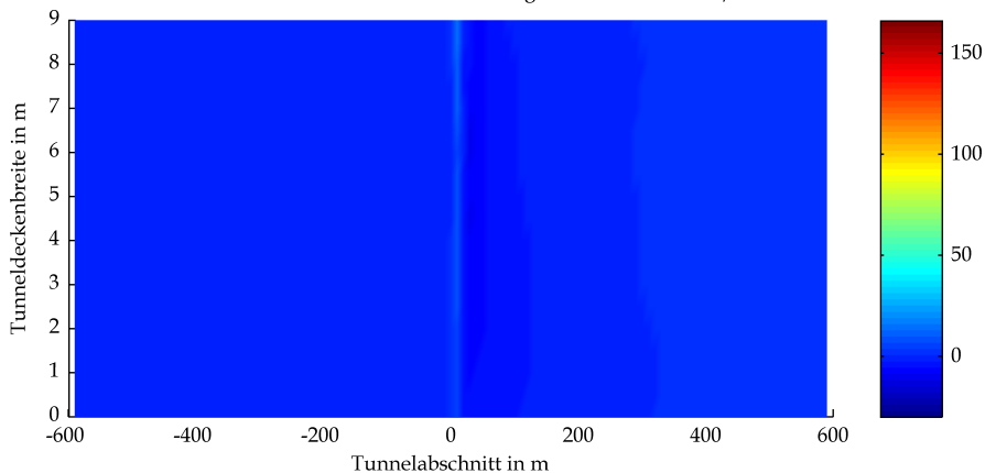
BAStBÜ Rechteck Mulde GV 20.6 owF Wärmestrahlung Tunneldecke in kW/m 2 bei t=2400s
