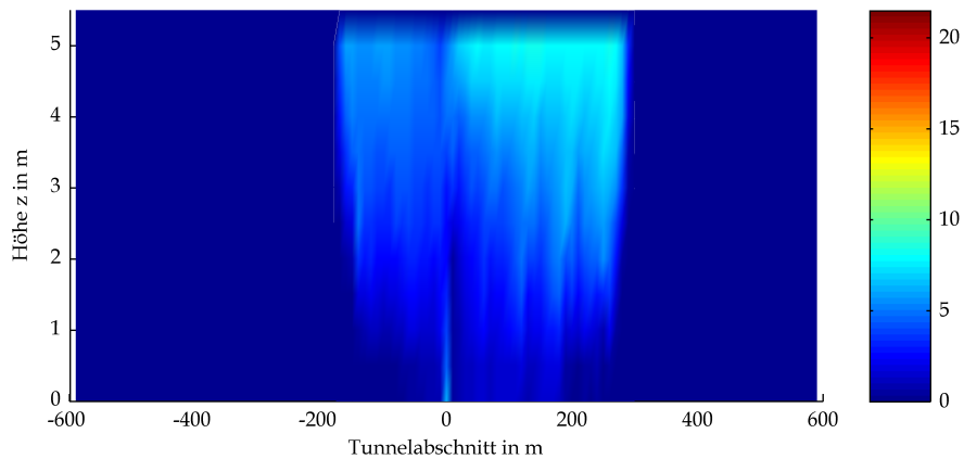
BAStBÜ Rechteck Mulde GV 20.6 owF Optische Dichte bei t=120s
