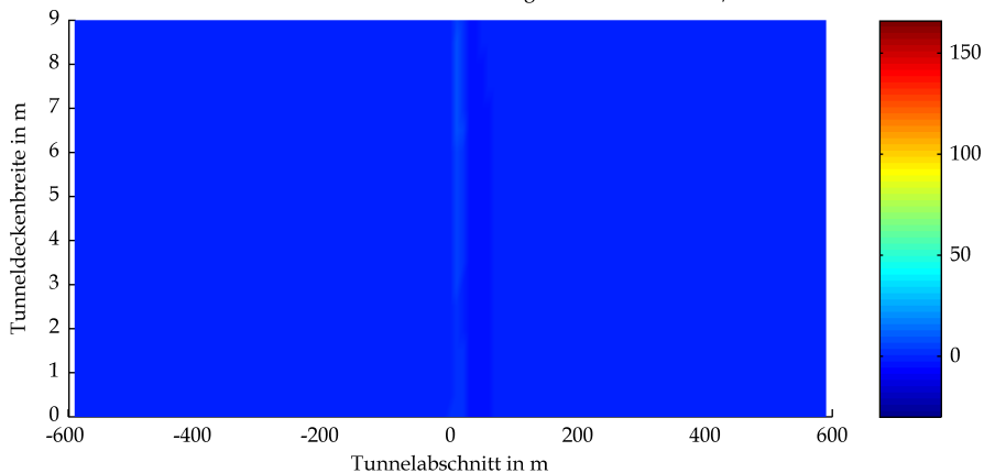
BAStBÜ Rechteck Mulde GV 20.6 owF Wärmestrahlung Tunneldecke in kW/m 2 bei t=3300s
