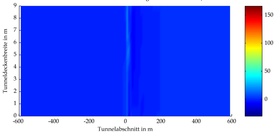
BAStBÜ Rechteck Mulde GV 20.6 owF Wärmestrahlung Tunneldecke in kW/m 2 bei t=2100s
