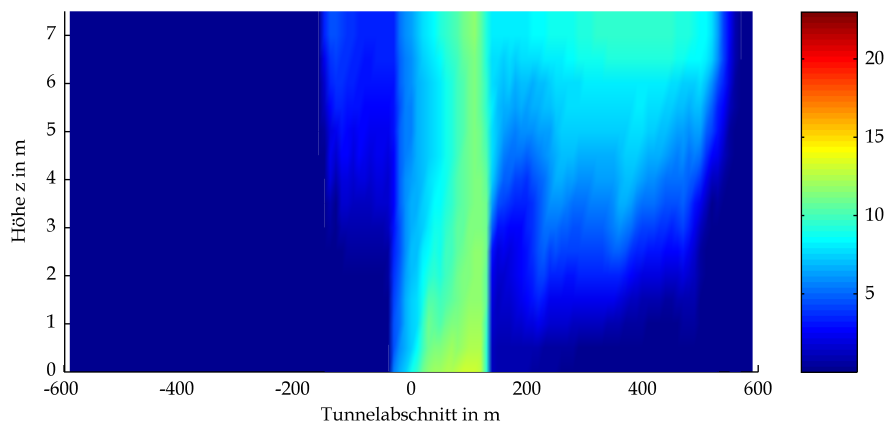
BASStBÜ Gewölbe Mulde RV 300 owF Optische Dichte bei t=120s
