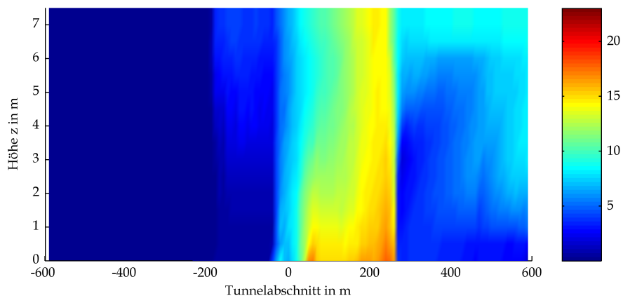
BASStBÜ Gewölbe Mulde RV 300 owF Optische Dichte bei t=180s
