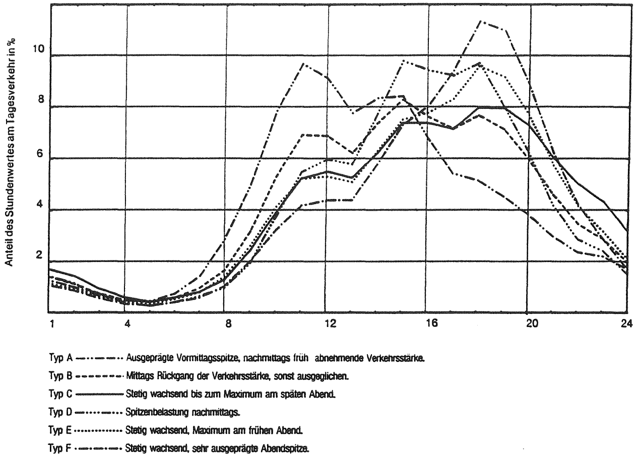
Bild 11: Tagesganglinien Sonntag
