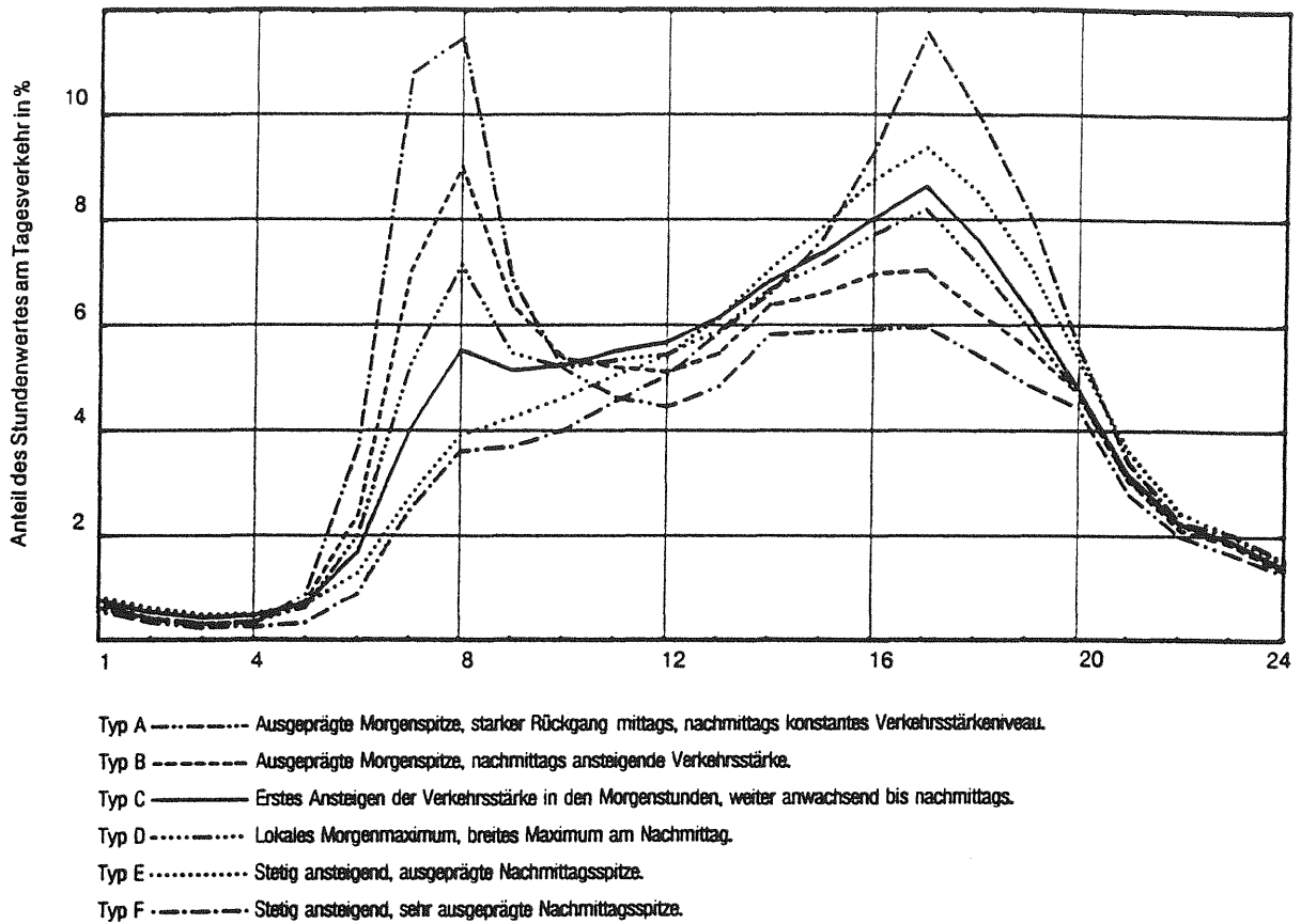
Bild 9: Tagesganglinien Freitag
