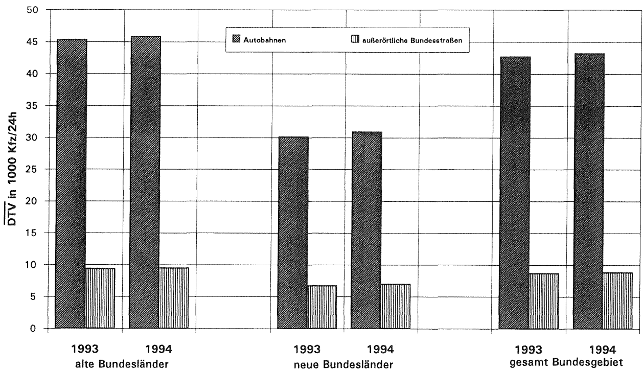
Bild 4: Verkehrsentwicklung auf Bundesautobahnen und außerörtlichen Bundesstraßen in der Bundesrepublik Deutschland
