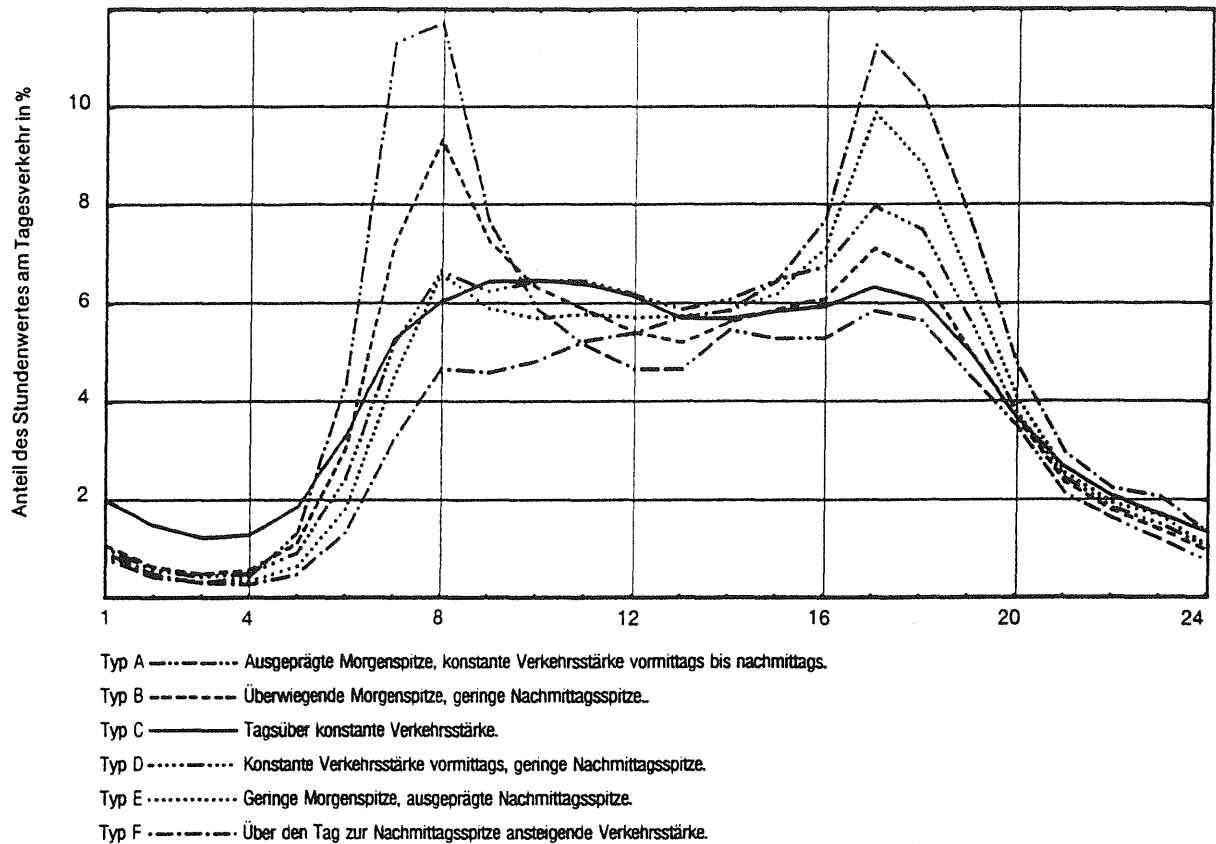
Bild 7: Tagesganglinien Montag
