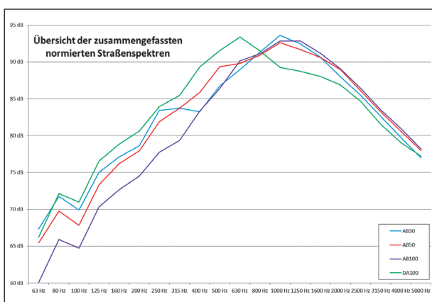
Bild A-1: Übersicht der zusammengefassten Straßenspektren (A-bewertet)
