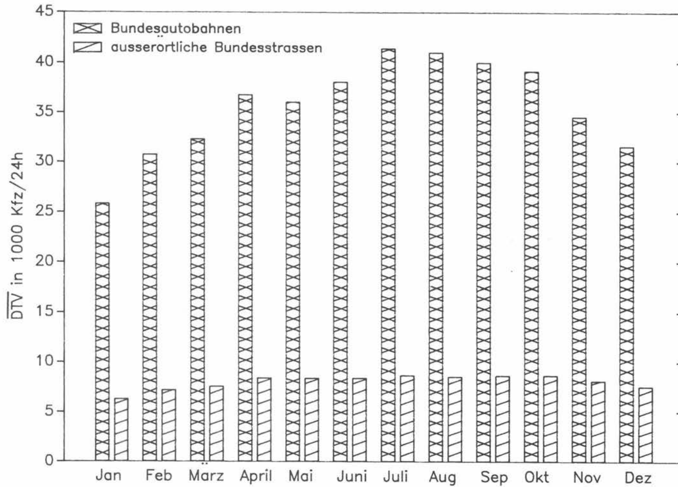
Bild 5: Mittlere DTV-Werte 1987 auf Bundesautobahnen und ausserörtlichen Bundesstrassen
