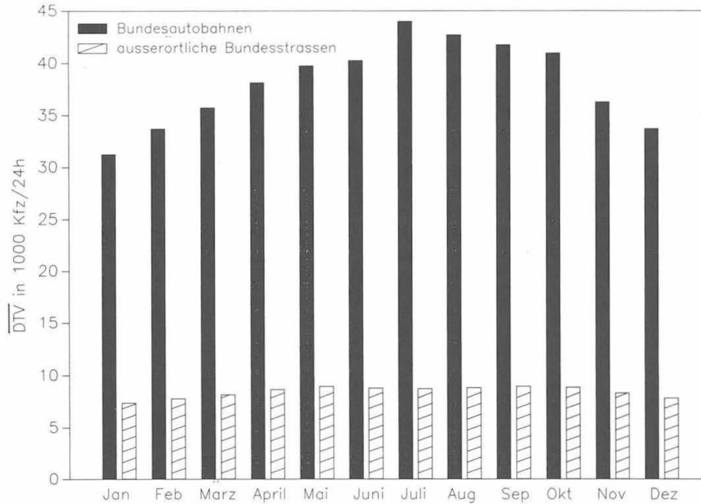
Bild 5: Mittlere DTW-Werte 1988 auf Bundesautobahnen und ausserörtlichen Bundesstrassen
