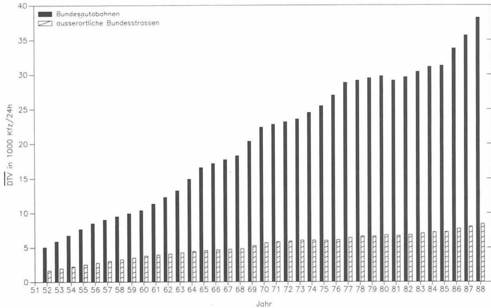
Bild 3: Verkehrsentwicklung auf Bundesautobahnen und ausserörtlichen Bundesstrassen
